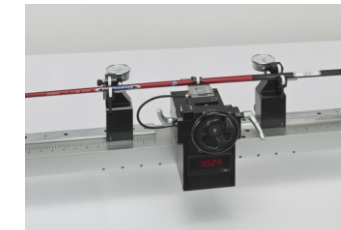
左右シャフト固定部の測定スパンを規格の中で設置し先端部・中央部・手元部の剛性値をシャフト軸周り全周にわたり測定が可能となりました。
