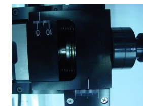
2mm/1回転ピッチのネジハンドルを廻しシャフトを圧縮 距離移動を与えます。
