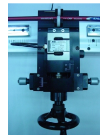
中央部にロードセルを備え水平に圧縮して荷負荷量を測れます
