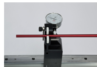
シャフトの偏平はダイヤルゲージで検知できます。
