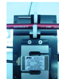
垂直方向に位置する2個のプーリーと抑えプーリーでシャフト軸を確実にホールドします。
